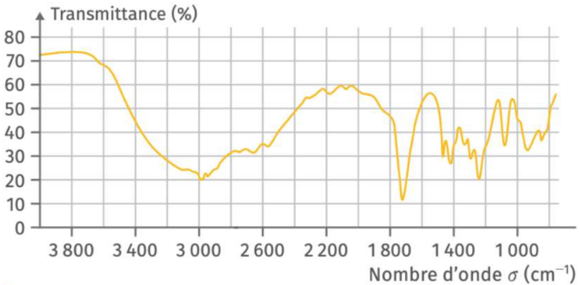
► Spectre IR des molécules du flacon n°2.
