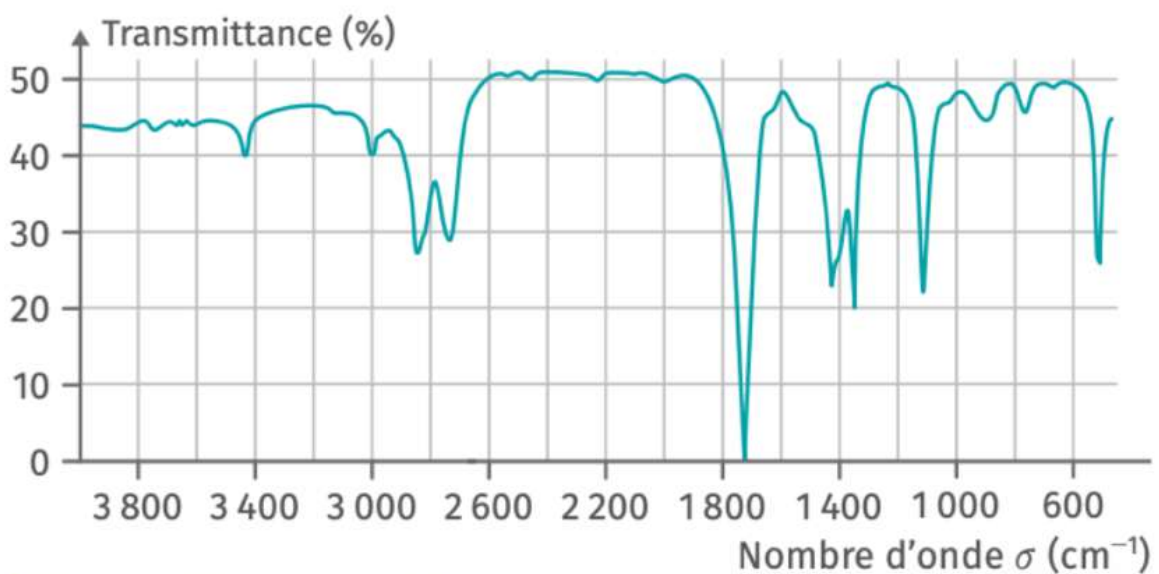
► Spectre IR des molécules du flacon n°3.
