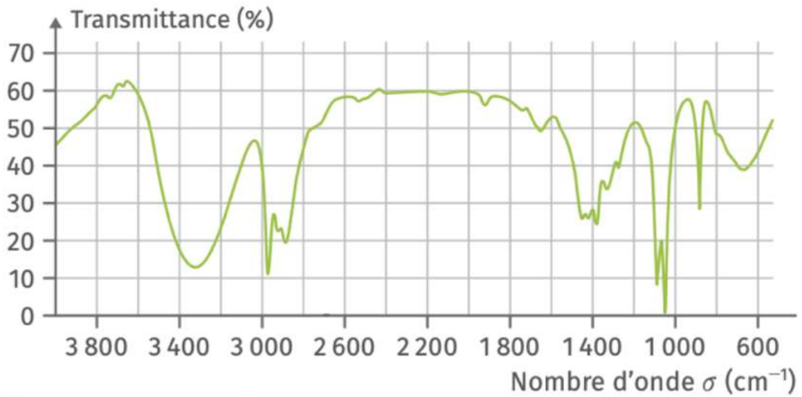
► Spectre IR des molécules du flacon n°1.
