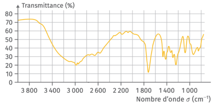
► Spectre IR des molécules du flacon n°2.
