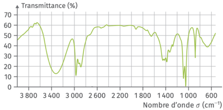
► Spectre IR des molécules du flacon n°1.
