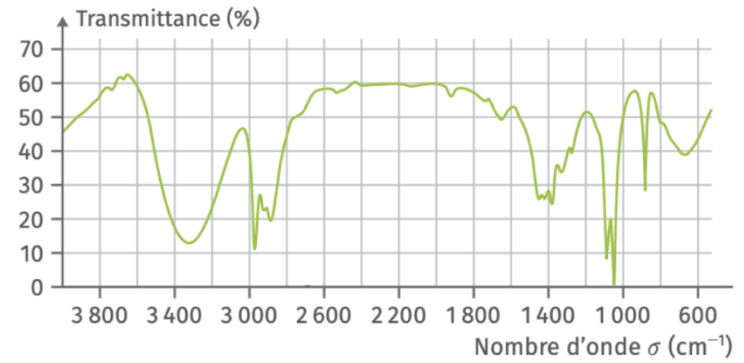
► Spectre IR des molécules du flacon n°1.
