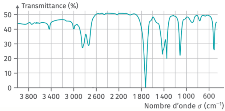
► Spectre IR des molécules du flacon n°3.
