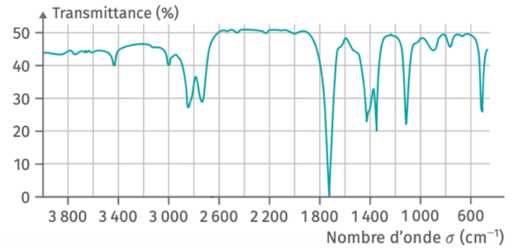
► Spectre IR des molécules du flacon n°3.
