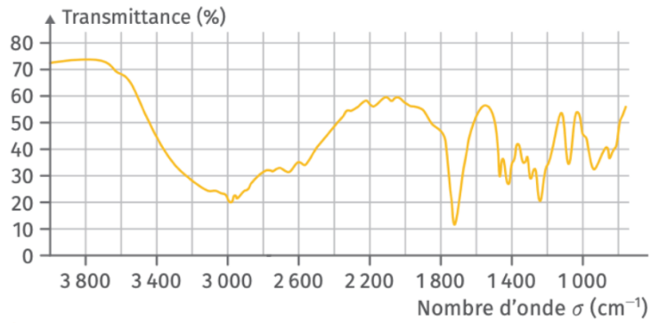
► Spectre IR des molécules du flacon n°2.
